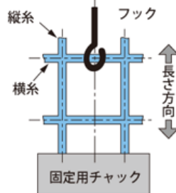
引掛強度試験 概略図 (横糸の試験の時)
