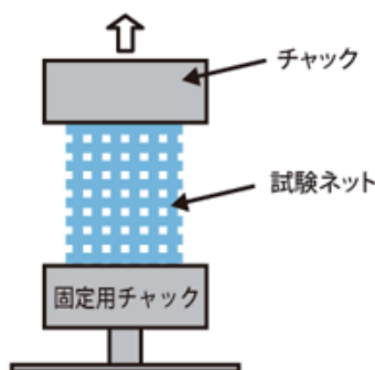
降伏点強度試験 概略図
