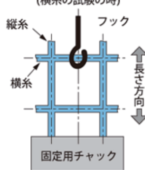
引掛強度試験 概略図 (横系の試験の時)
